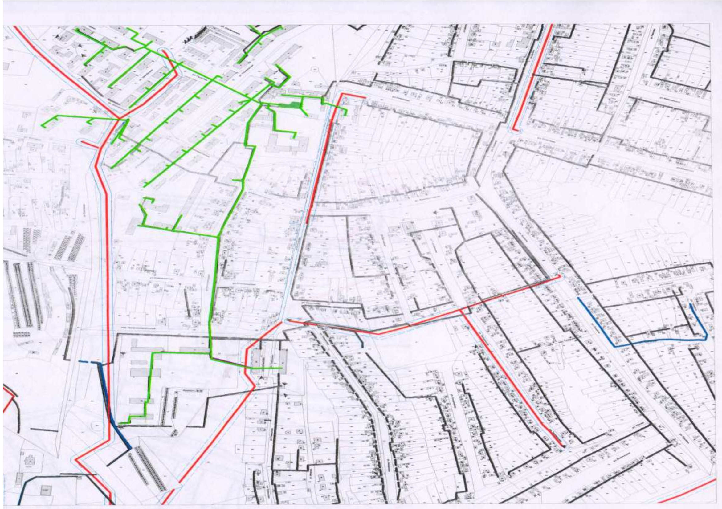
Рисунок 1.3.2.25 - Схема тепловых сетей котельной №1 п.г.т. Алексеевка
