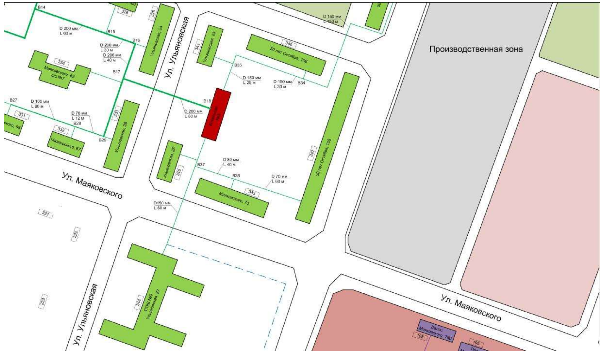
Рисунок 1.3.2.6 - Схема тепловых сетей котельной №3 г. Кинель
