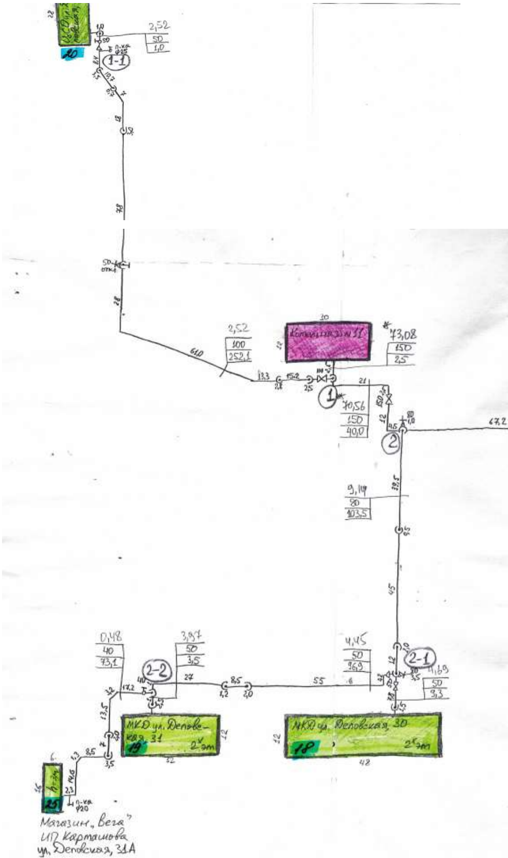
Рисунок 1.3.2.14 - Схема тепловых сетей котельной №11 г. Кинель
