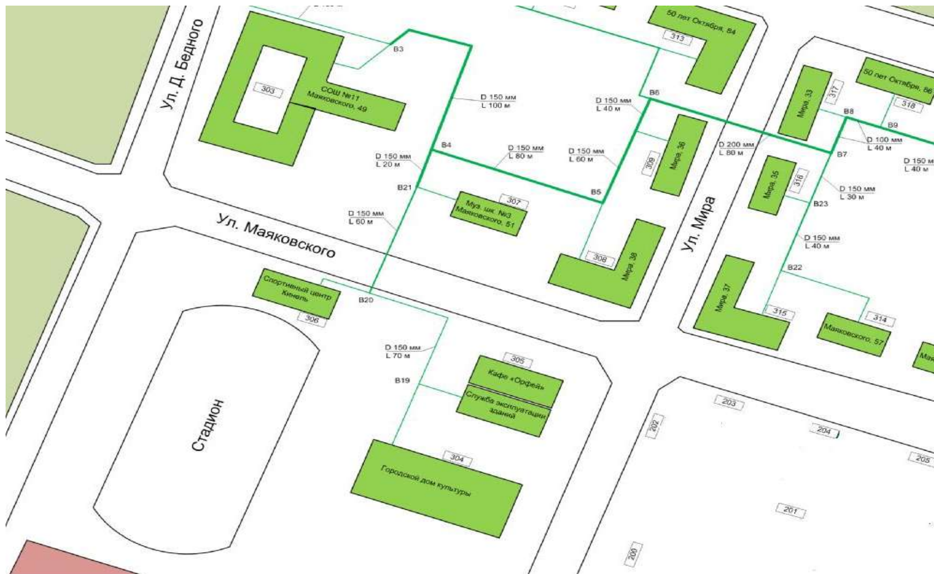
Рисунок 1.3.2.4 - Схема тепловых сетей котельной №3 г. Кинель
